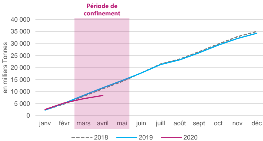
Production cumulée de granulats en Occitanie
