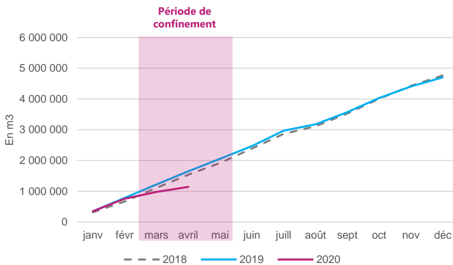
Production cumulée de béton prêt à l'emploi en Occitanie
